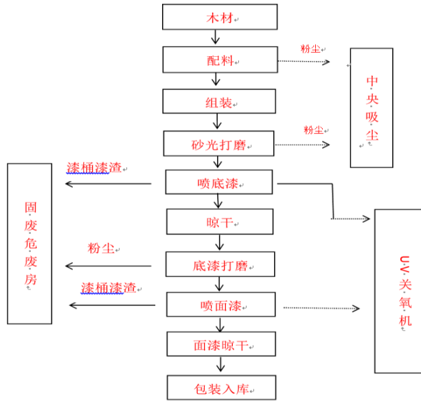
图 1.生产工艺流程及产排污环节
